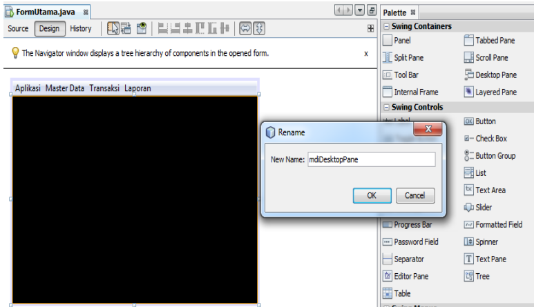
Gambar 1. 14 Menambahkan Desktop Pane Pada Design Form Utama
